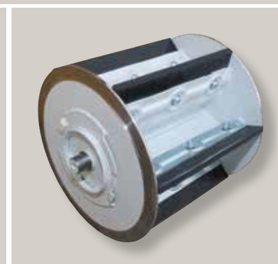
Rotor de la tolva receptora CA 20, equipado con paletas de goma.
